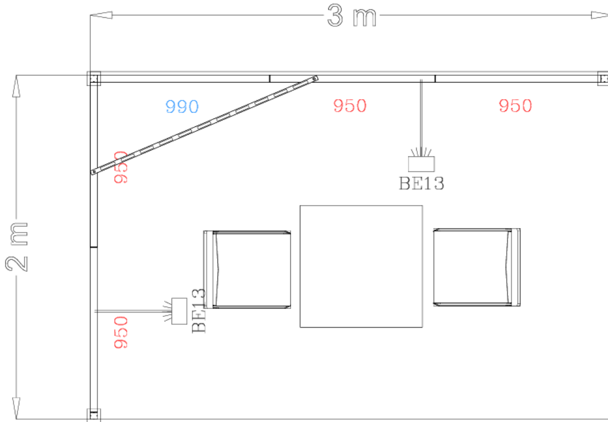
Draufsicht/Top View
